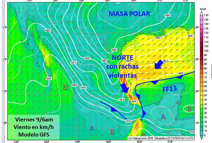
Modelo GFS. Mié 07/12/2016, 00 UTC. Pronóstico para el Vie 09/12/2016, 12 UTC (H+60) Viento a 10m (Kmh) / Presión al nivel del mar (hPa)
